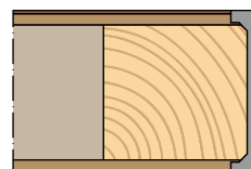
Zichtbare aangegoten kantlat - PU
