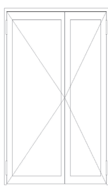
Porte 2 vantaux tiercé
