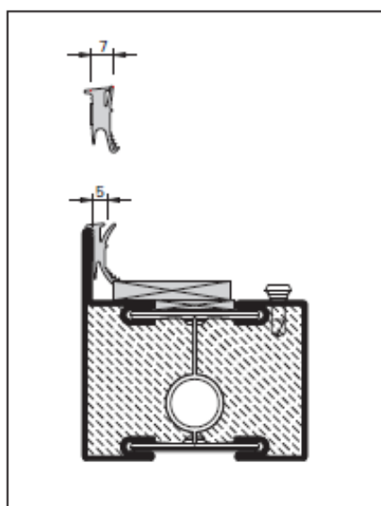
Montage joint côté aile fixe
