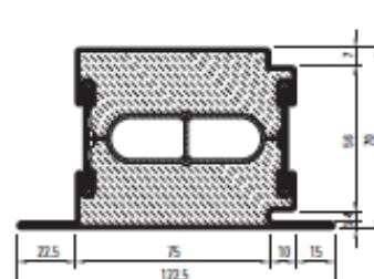
630.115.C4 630.115.C4 Z
