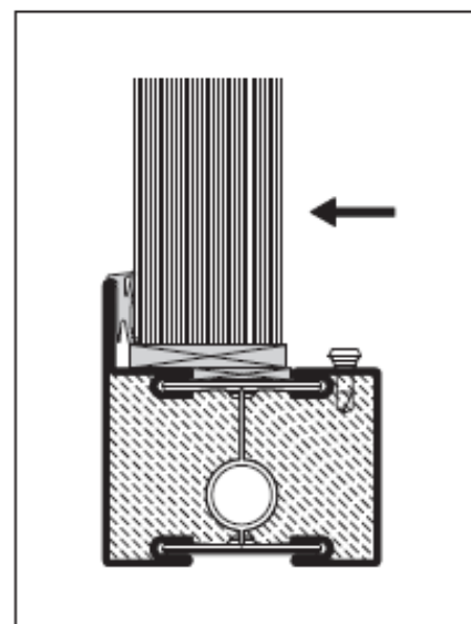
Pose du vitrage
